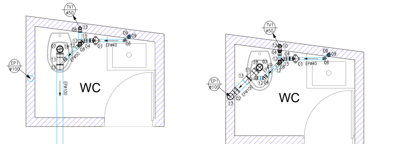
DETALHE 02 - WC SUPERIOR
