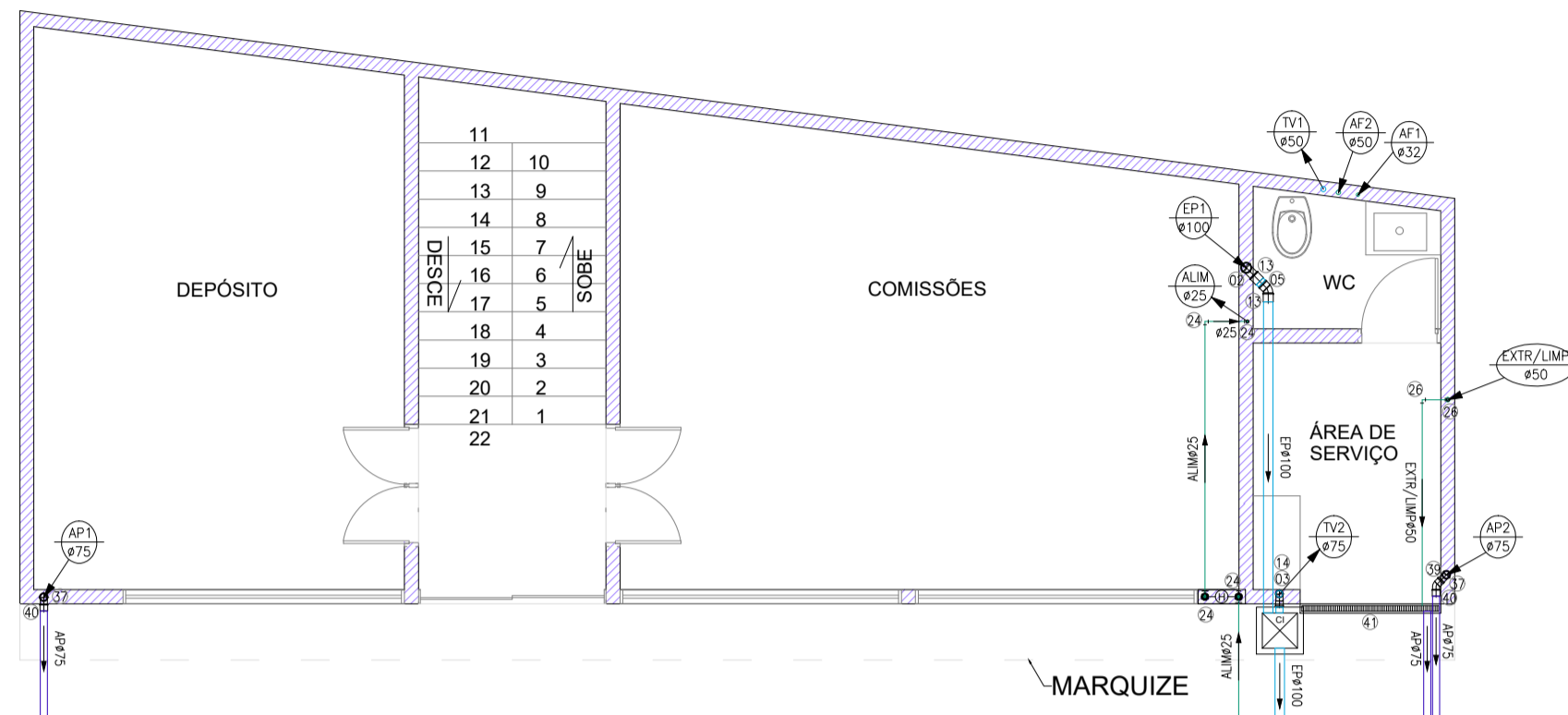
PLANTA BAIXA PAVIMENTO TÉRREO
